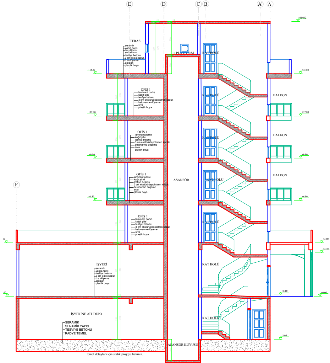
B-B KESİTİ Ö:1/50
